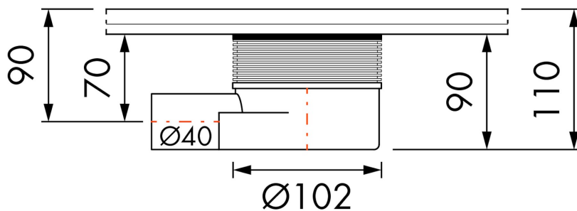
Easy Drain® EDMSI-6, WS-50 mm
