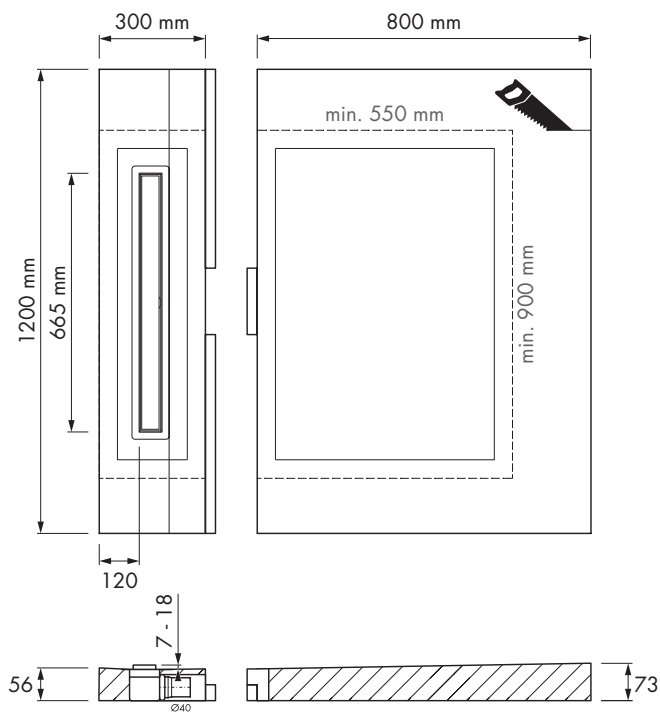
Showerboard Compact / Modulo M1
